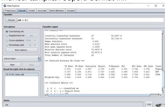
Gambar 10 Tampilan Hasil Analisa Classify
