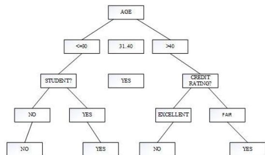
Gambar 2. Model Pohon Keputusan
