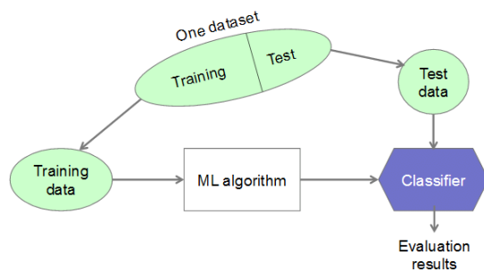
Gambar 2. Data Train dan Data Testing
