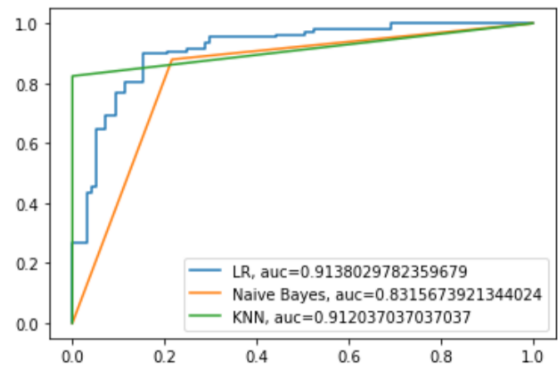
Gambar 12. Nilai AUC dari ketiga algoritma
