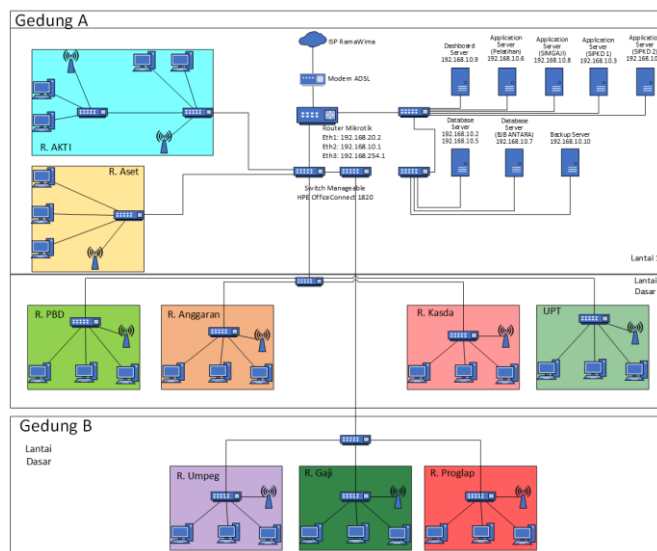
Gambar1. Skema Jaringan BPKAD Kab. Bogor
