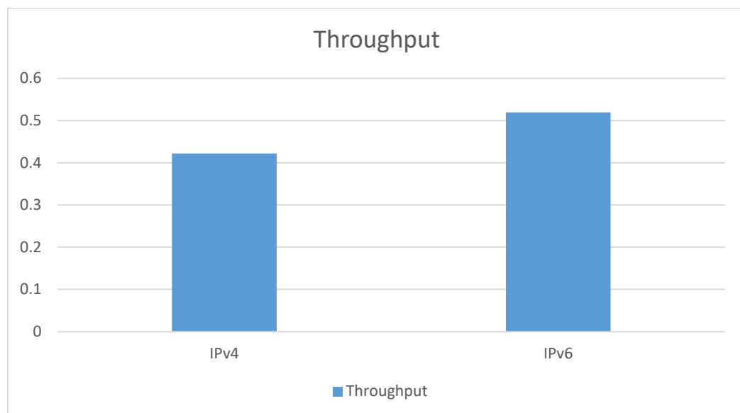
Gambar 3. Grafik perbandingan rata-rata Throuput dengan file 30 MB
