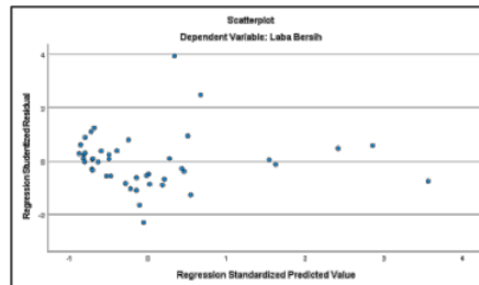
Gambar 2. Grafik Scatterplot Uji Heteroskedastisitas
