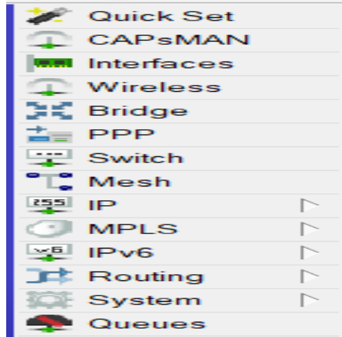
Gambar 17. Tampilan Queue
