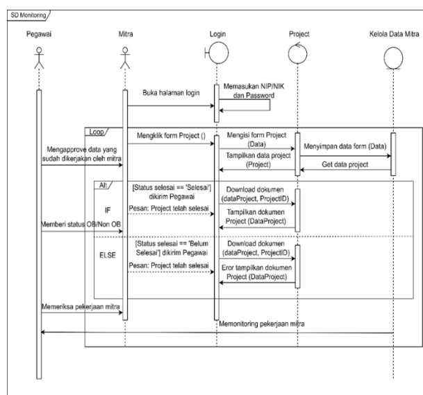
Sequence Diagram dipergunakan untuk menggambarkan kelakuan objek di use case.
