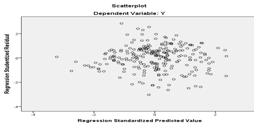
Gambar 4.2 Uji Heteroskedastisitas
