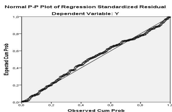
Gambar 4.1 Uji Normalitas
