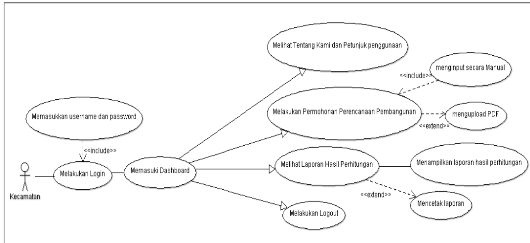
Gambar 8. Use Case Diagram Rancangan Usulan Penentuan Prioritas Perencanaan Pembangunan Daerah Bagian User
