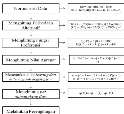
Gambar 1. Bagan Perhitungan Metode Promethee
