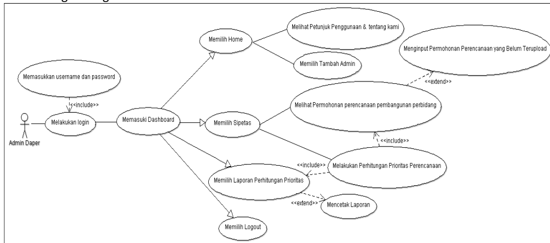
Gambar 9. Use Case Diagram Rancangan Usulan Penentuan Prioritas Perencanaan Pembangunan Daerah Bagian Admin
