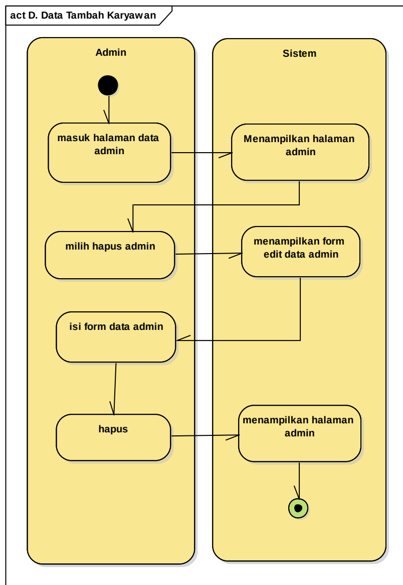
Gambar IV.6 Diagram Activity Tambah Karyawan
