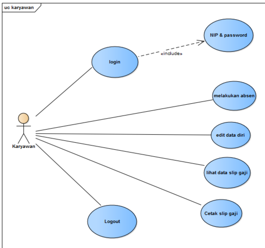
Gambar IV.1 Usecase Diagram Karyawan
