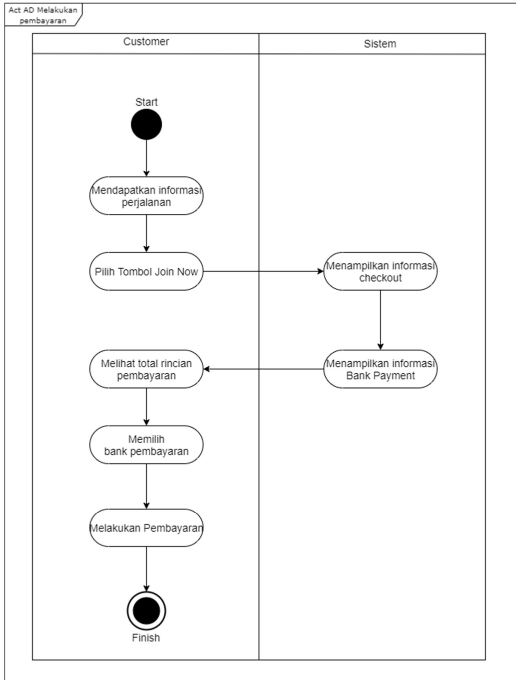
Gambar IV.7 Rancangan Diagram Aktivitas Melakukan Pembayaran
