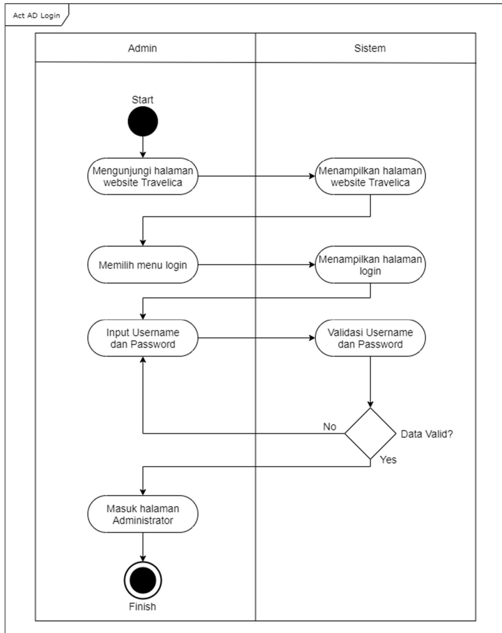
Gambar IV.2 Rancangan Diagram Melakukan Login
