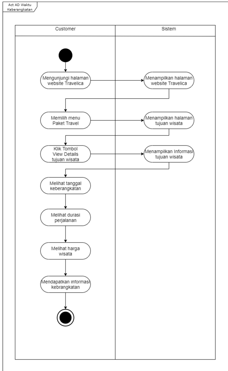
Gambar IV.4 Rancangan Diagram Aktivitas Waktu Keberangkatan
