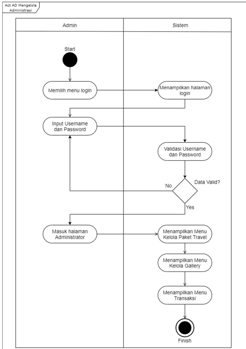
Gambar IV.9 Rancangan Diagram Aktivitas Mengelola Administrasi
