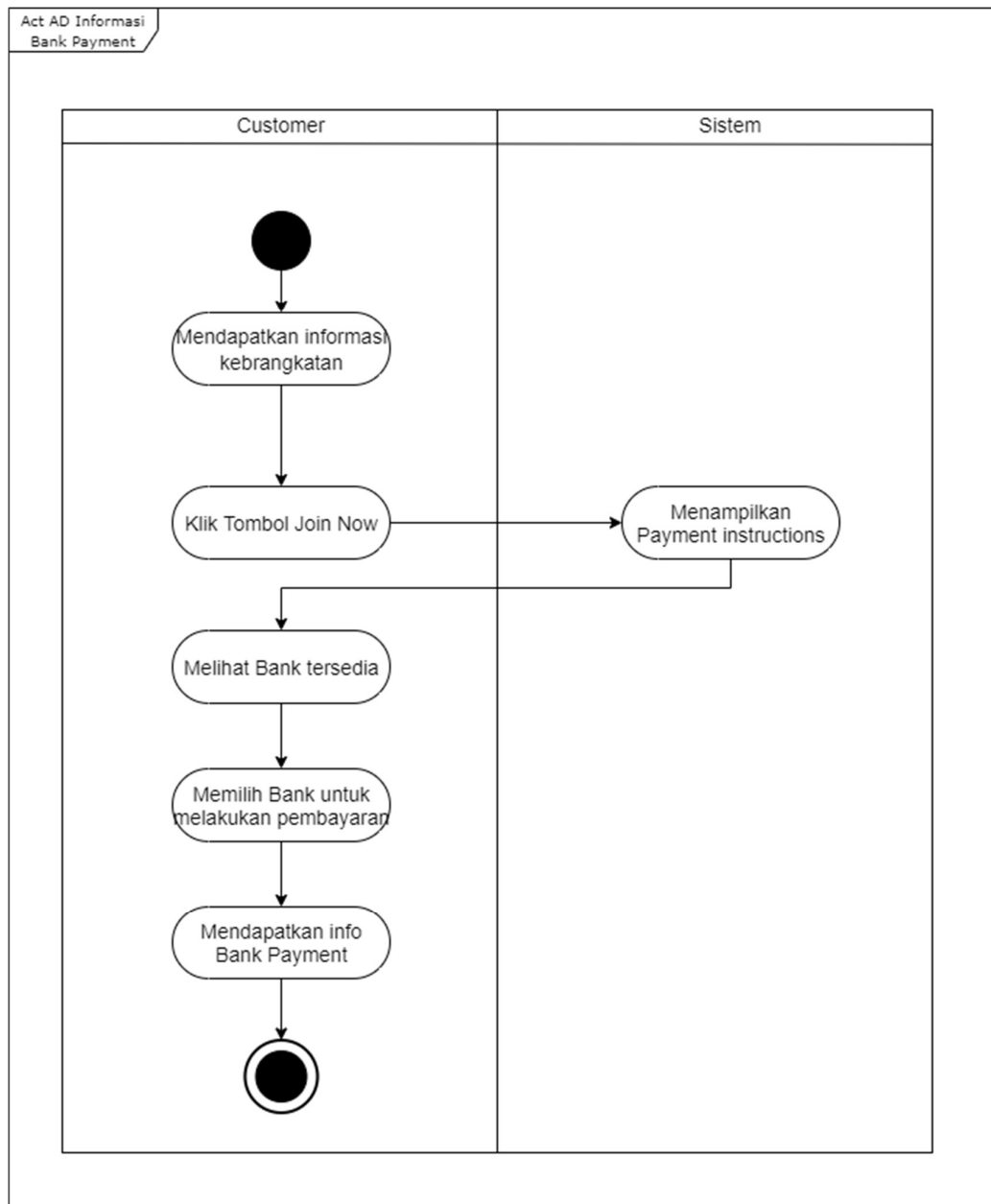
Gambar IV.6 Rancangan Diagram Aktivitas Melihat Informasi Bank Payment
