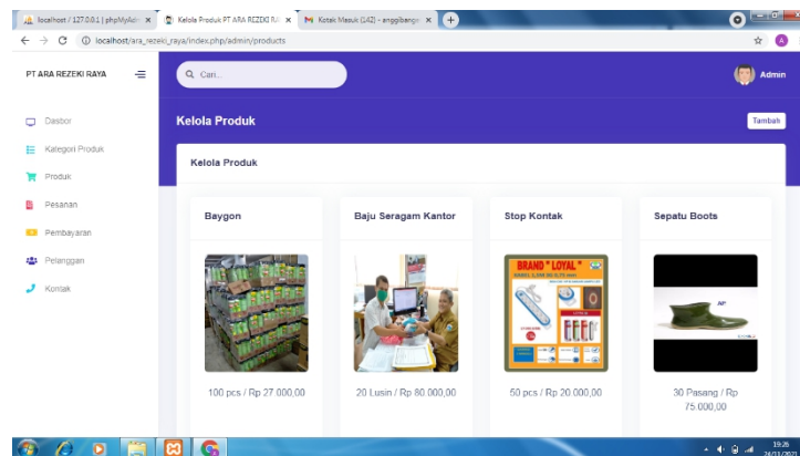
Gambar III.10.5 Halaman Produk
