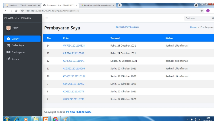
Gambar III.10.7 Halaman Pembayaran
