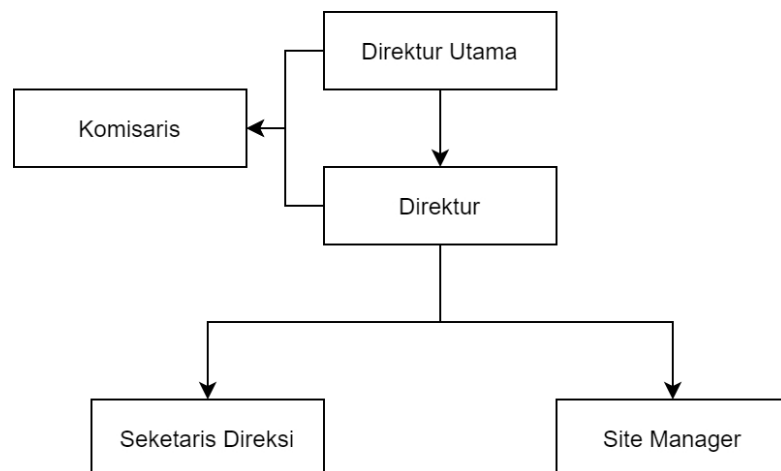
Gambar III.3 Struktur Organisasi
