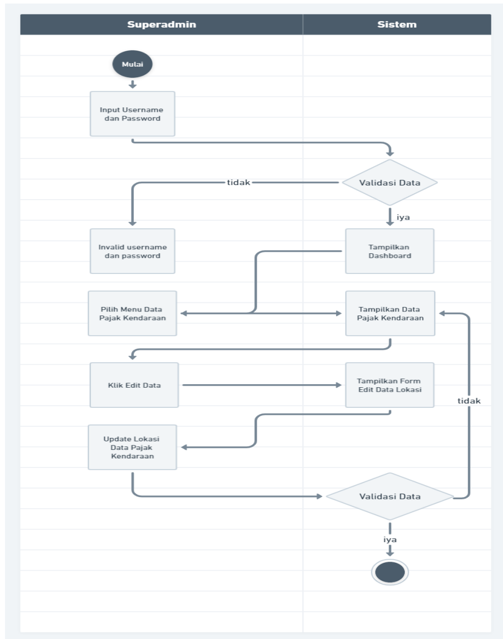
Gambar 4.6 Activity Diagram Admin Update Lokasi Kendaraan
