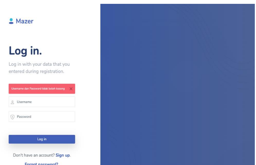
Gambar 4.40 Login Jika Username Dan Password Kosong
