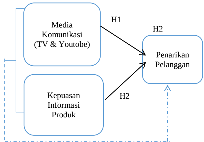
Gambar 2. Kerangka Berfikir
