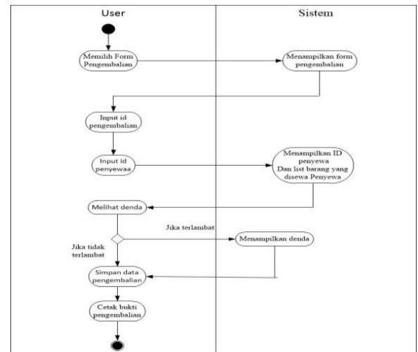
Gambar 4. Activity Diagram Pengembalian alat gunung
