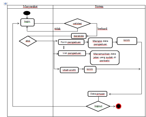
Sumber : Hasil Penelitian (2021) Gambar 5. Activity Diagram Masyarakat Sebagai pemetaan basis data, maka digambarkan dengan menggunakan ERD, yaitu :
