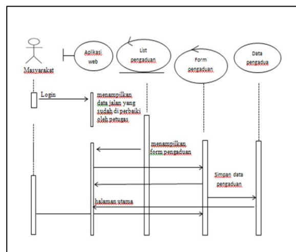
Gambar 11. Rancangan Sequence Diagram Masyarakat
