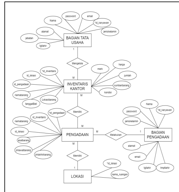
Gambar 7. Rancangan ERD
