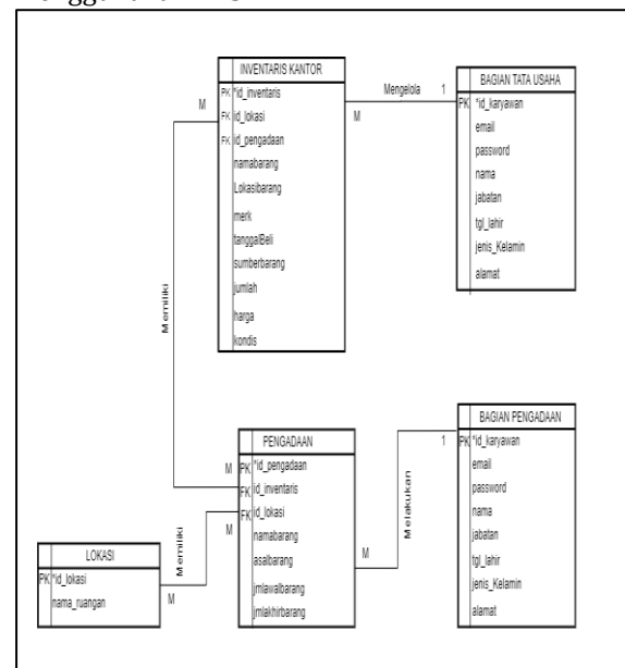
Gambar 8. Rancangan LRS
