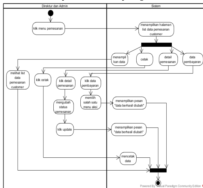
Gambar 7. Activity Diagram Pemesanan Direktur dan Admin.
