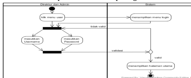
Gambar 4. Activity diagram login direktur dan admin.
