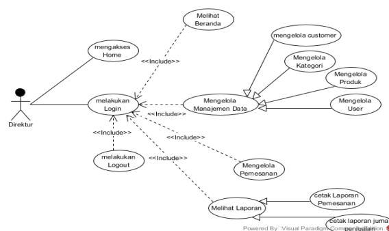
Gambar 1. Use Case Diagram Direktur
