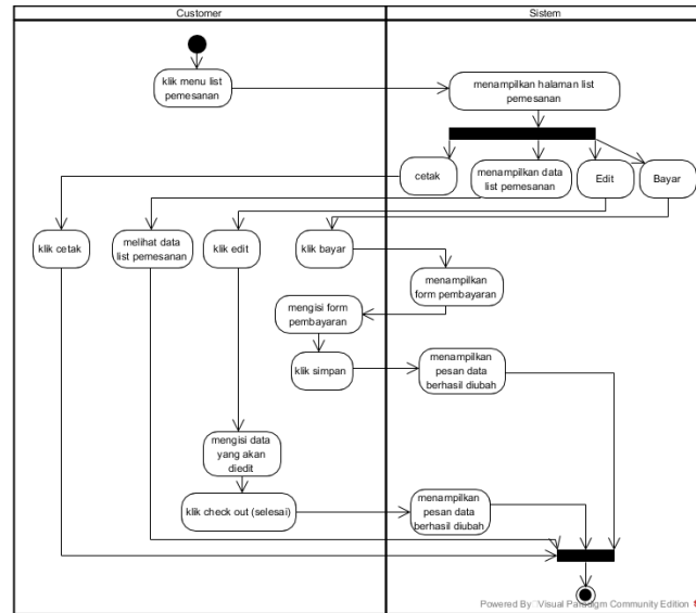
Gambar 11. Activity Diagram Menu List Pemesanan pada Customer.
