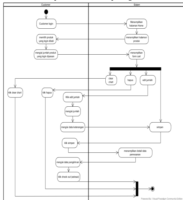
Gambar 10. Activity Diagram Pemesanan pada Customer.
