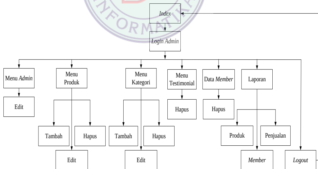
Gambar III.51. Struktur Navigasi Admin
