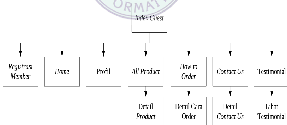
Gambar III. 49. Struktur Navigasi Pengunjung
