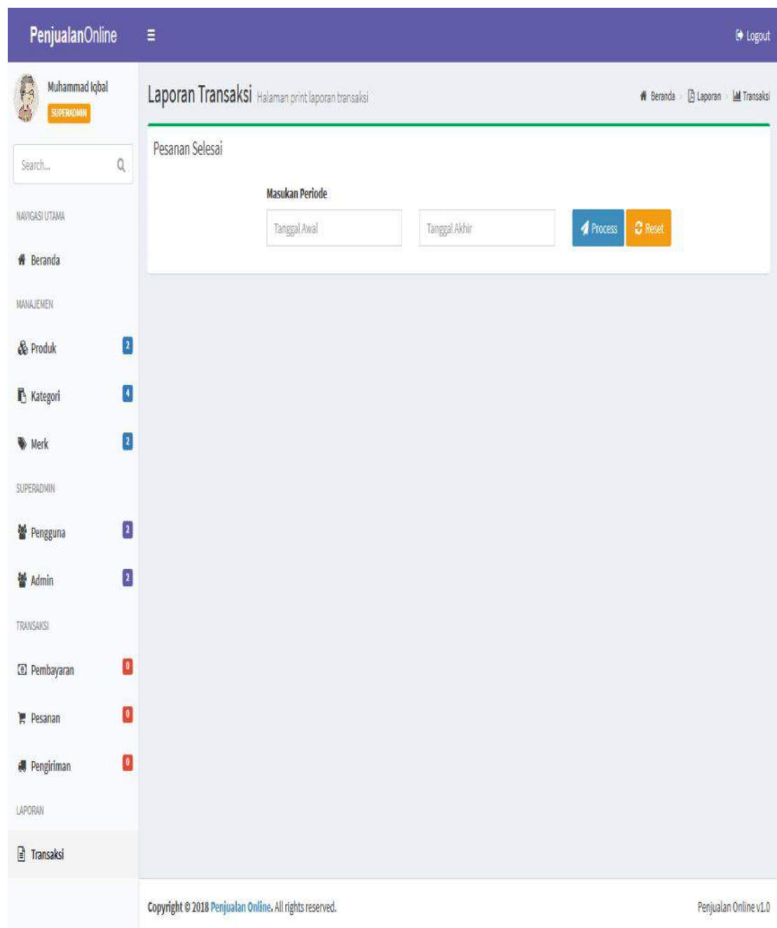
Gambar III. 14 Halaman Antar Muka Laporan Transaksi Admin
