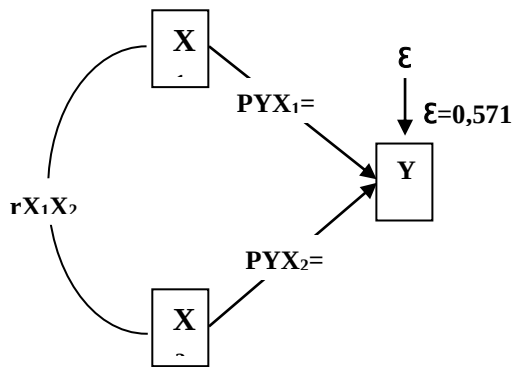
Gambar 2. Struktur Analisis Jalur
