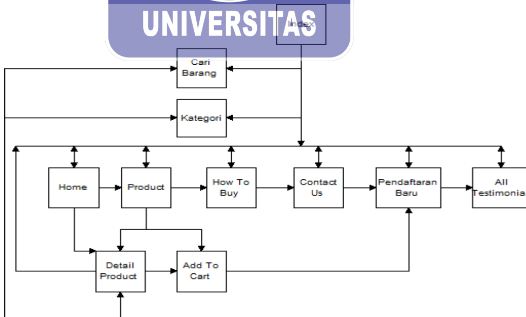
Gambar III.57. Struktur Navigasi Pengunjung
