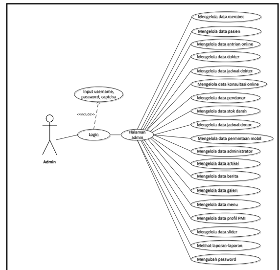
Gambar 1. Use Case Diagram Mengelola Halaman Admin
