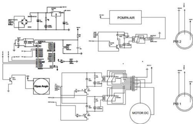
Gambar 2. Rangkaian Alat
