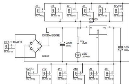
Gambar 3. Rangkaian Catu Daya
