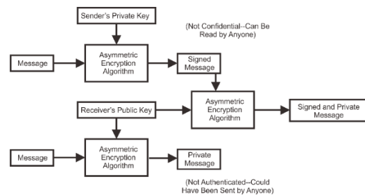
Gambar 6 Enkripsi Asimetris
