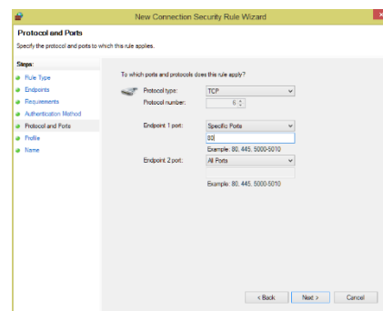
Gambar 14 Menentukan Protokol dan Port
