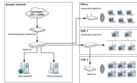
Gambar 2. Topologi jaringan usulan
