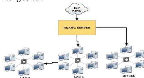
Gambar 1. Topologi jaringan lama
